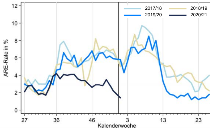
Abb. 1: Vergleich der für die Bevölkerung in Deutschland geschätzten ARE-Raten (in Prozent) in den Saisons 2017/18 bis 2020/21, 1. KW 2021. Der schwarze, senkrechte Strich markiert den Jahreswechsel.
