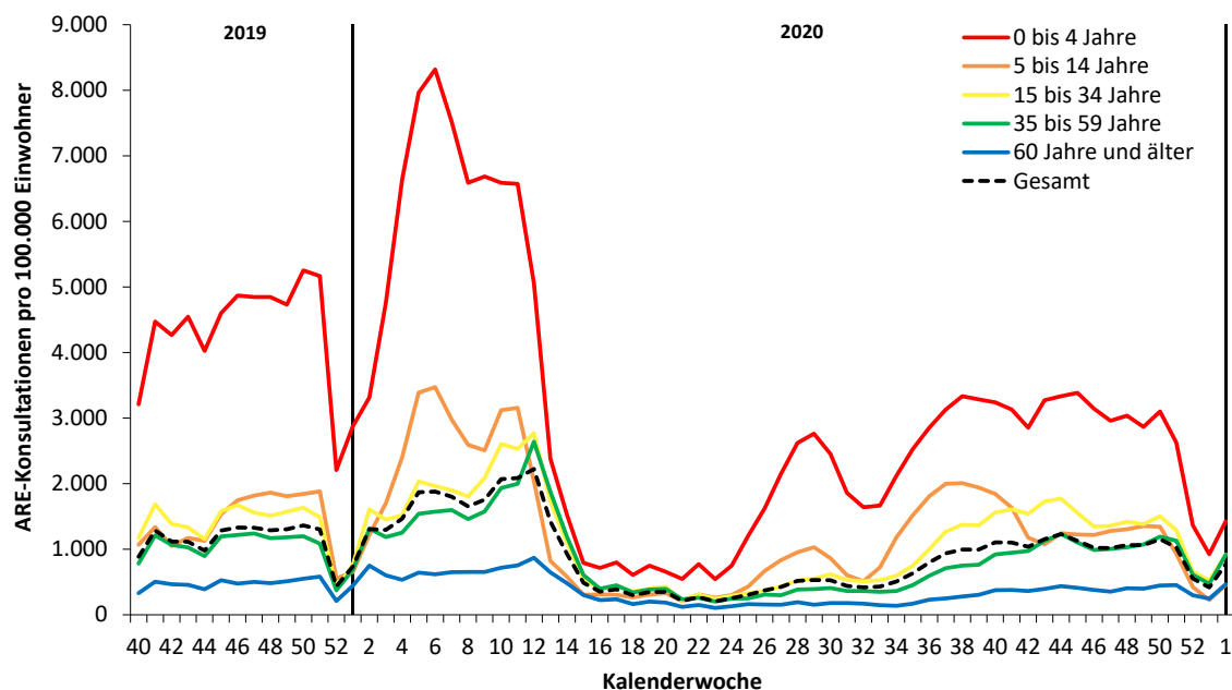
Abb. 3: Werte der Konsultationsinzidenz von der 40. KW 2019 bis zur 1. KW 2021 in fünf Altersgruppen und gesamt in Deutschland pro 100.000 Einwohner in der jeweiligen Altersgruppe. Der senkrechte Strich markiert die 1. KW des Jahres.
