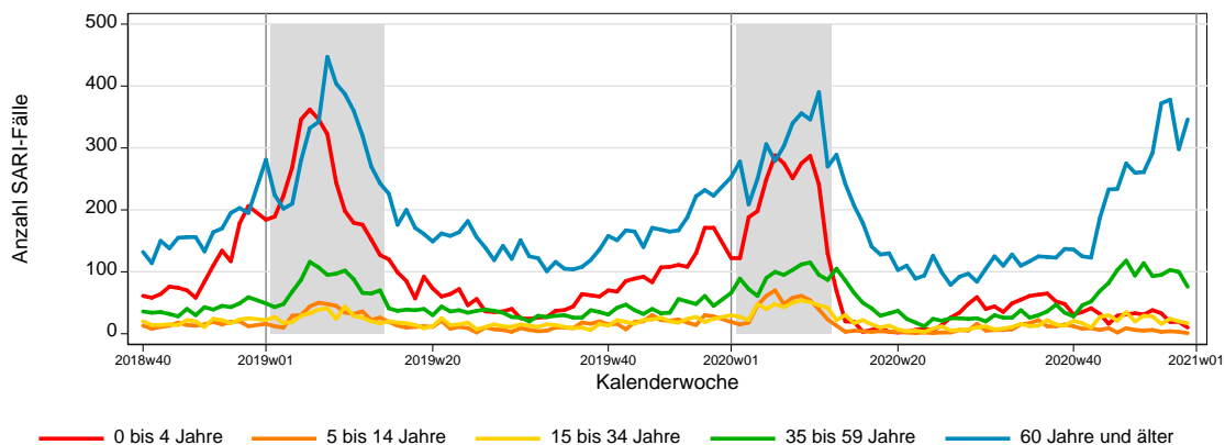
Abb. 4: Wöchentliche Anzahl der SARI-Fälle (ICD-10-Codes J09 – J22) mit einer Verweildauer bis zu einer Woche von der 40. KW 2018 bis zur 53. KW 2020, Daten aus 72 Sentinelkliniken. Der senkrechte Strich markiert jeweils die 1. KW des Jahres, der Zeitraum der Grippewelle ist grau hinterlegt.
